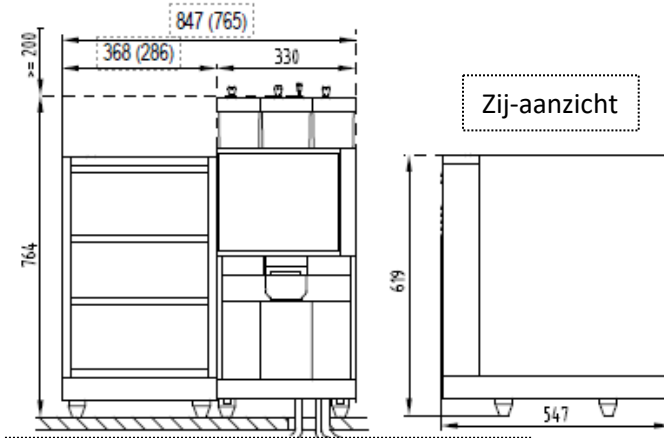
Koppenswarmer (links, rechts) Vereist: extra wandcontactdoos Smalle uitvoering : Vermogen = tot 160 W / Gewicht = 30Kg Brede uitvoering : Vermogen = tot 170 W / Gewicht = 34Kg
