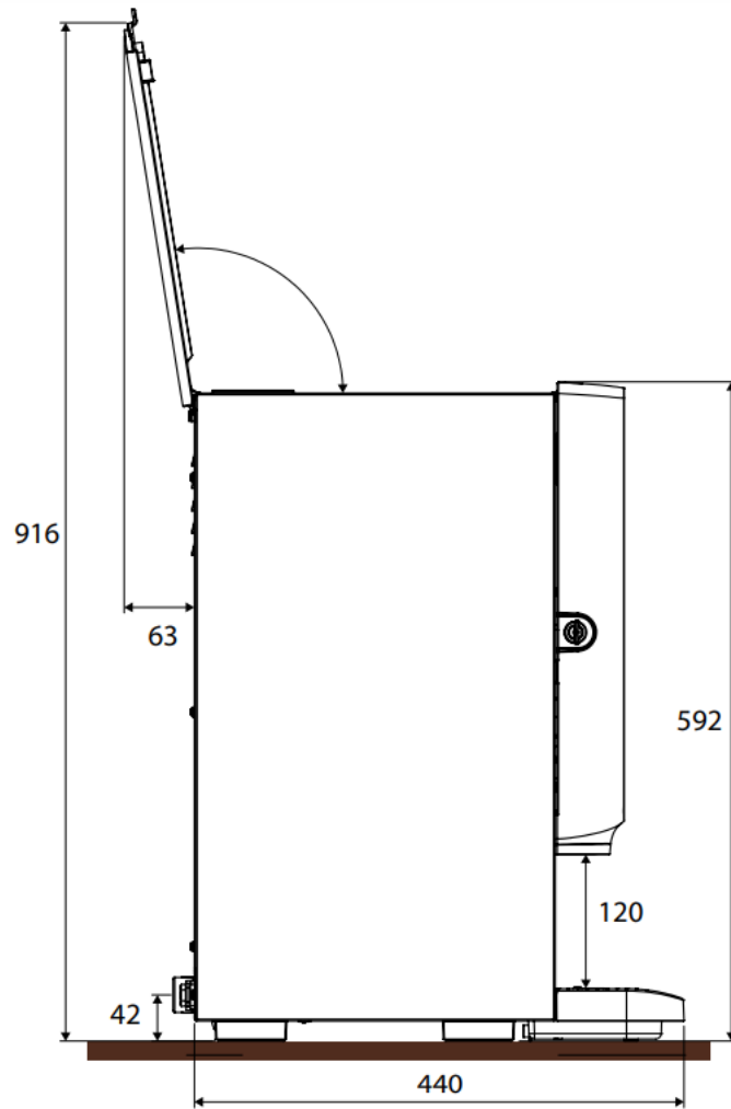
Zijkant met geopend bovendeksel (+80 mm ruimte aan de achterzijde)
